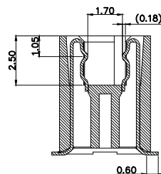
SECTION A-A Scale 2:1
